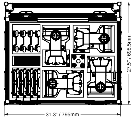
Top view, lid open
