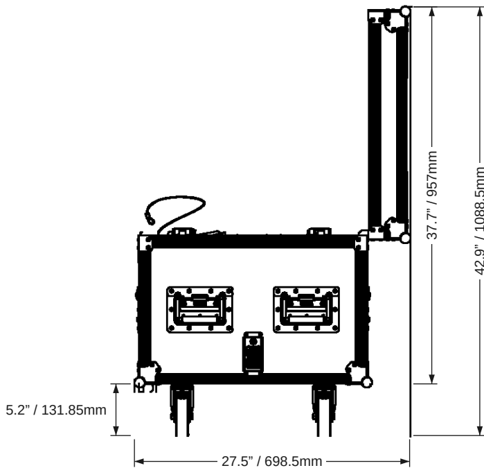
End view, lid open
